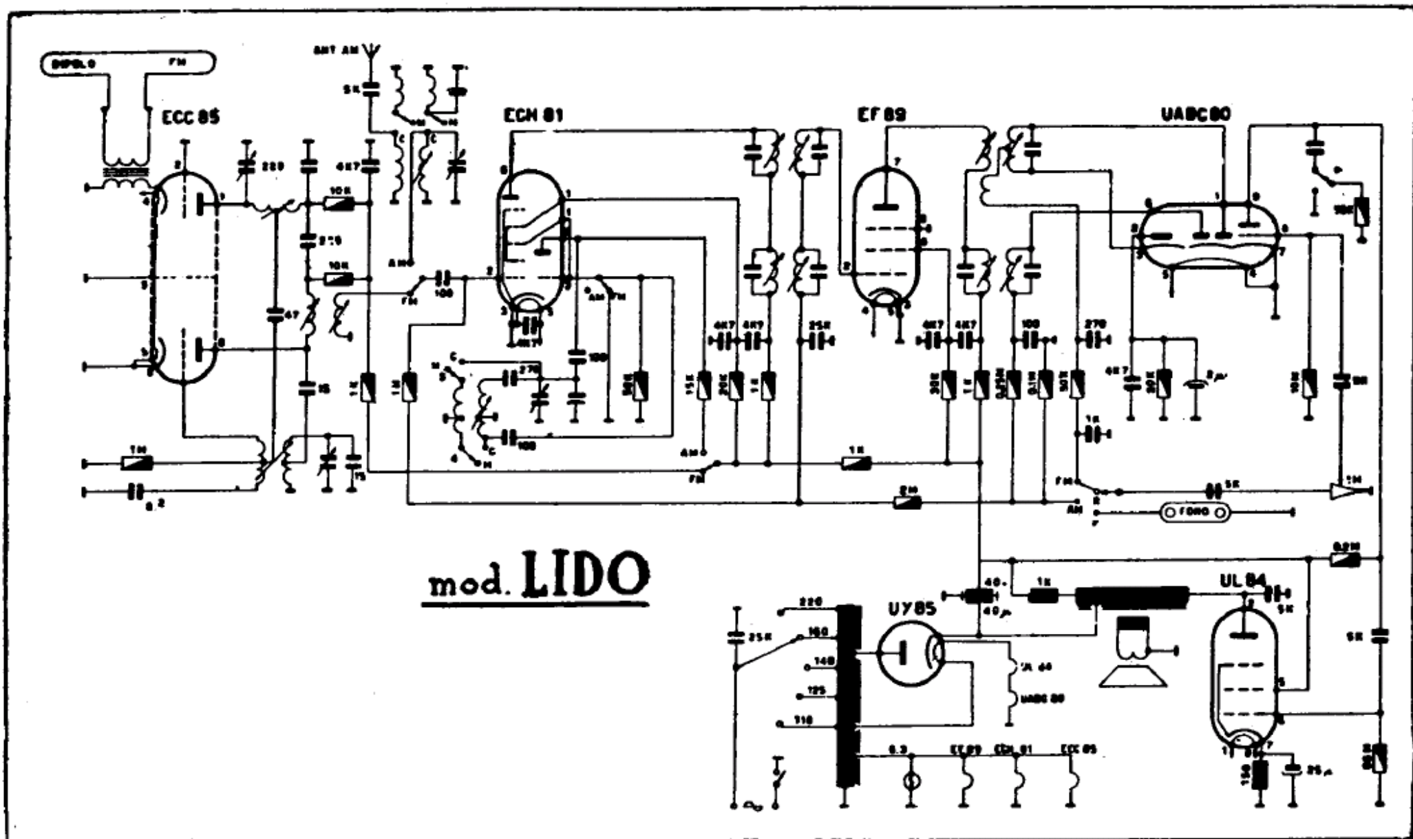
WINNER - Mod. LIDO. Apparecchio AM/FM, con gamma onde medie da 190 a 580 metri, e banda onde ultracorte da 87,5 a 100,5 Mc/s. Medie frequenze a 468 kc/s e a 10,7 Mc/s. Resa d'uscita 2,5 watt. Consumo 38 watt.
